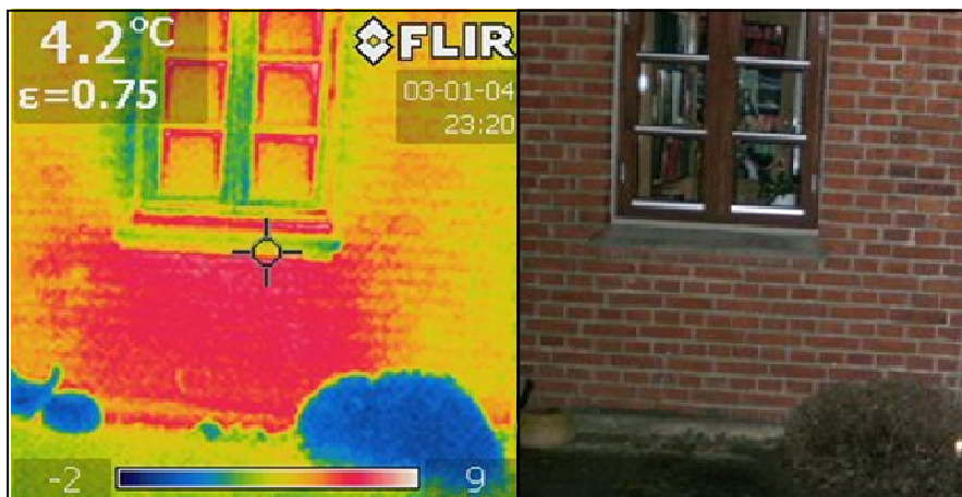
Eksempel på termograferingsfoto med tilhørende digitalfoto. Termograferingsfotoet viser, at der er varmeudslip under vinduet, hvilket ikke kan ses på det digitale foto. Fortsættes →
